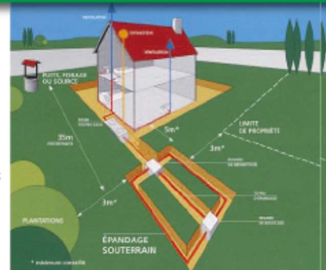
Épandage souterrain en sol naturel
